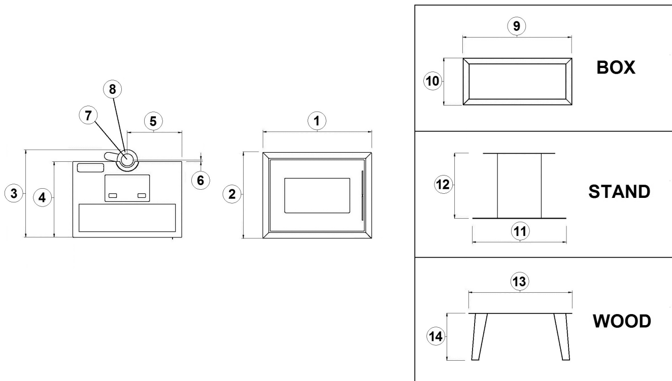
Fig. 16 - Dimensioni generali: MODO AT
