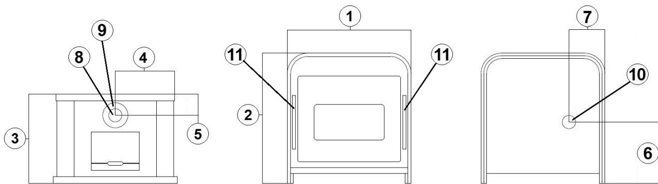
Fig. 14 - Dimensioni generali: FRAME 3 UP
