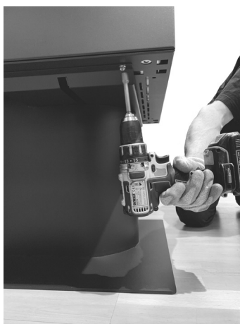
Fig. 18 - Fissaggio piedistallo
