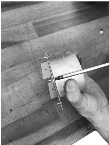
Fig. 31 - Fissare flangia al raccordo
