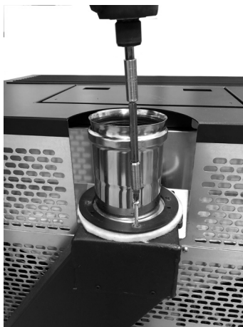
Fig. 42 - Svitare lo scarico
