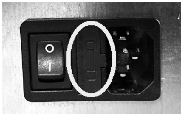
Fig. 66 - Sportellino con i fusibili da rimuovere
