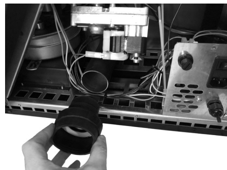
Fig. 46 - Rimuovere raccordo siliconico
