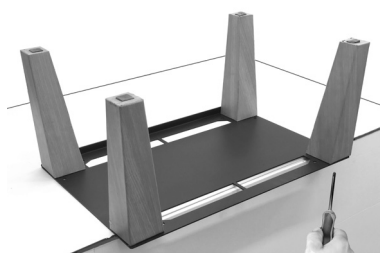
Fig. 20 - Fissare gambe alla base
