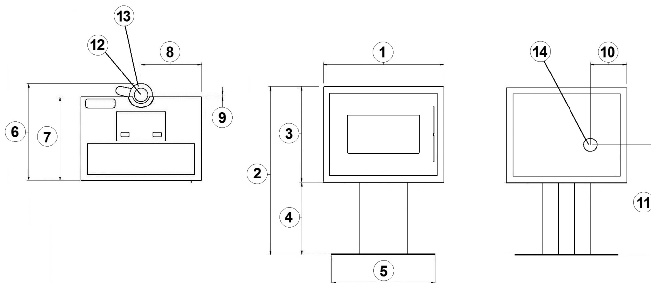
Fig. 15 - Dimensioni generali: QUASIMODO 3 UP
