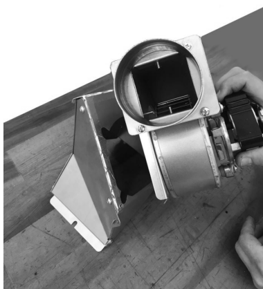
Fig. 35 - Fissare ventilatore al carter
