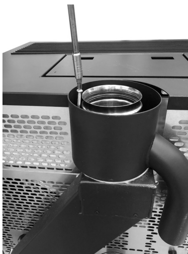
Fig. 45 - Fissare tubo il concentrico
