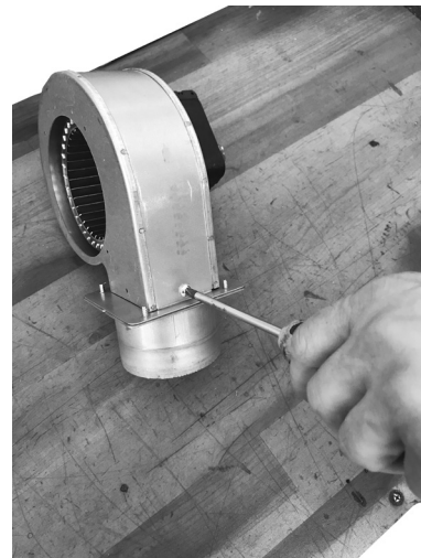
Fig. 33 - Fissare con viti
