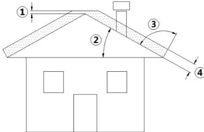
Fig. 3 - Tetto inclinato
