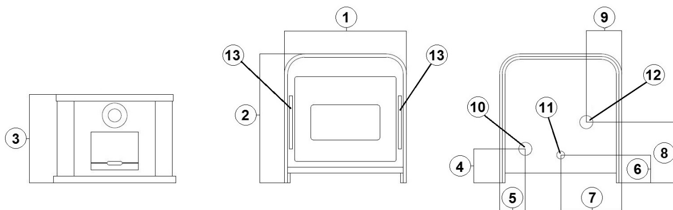
Fig. 13 - Dimensioni generali: FRAME 3
