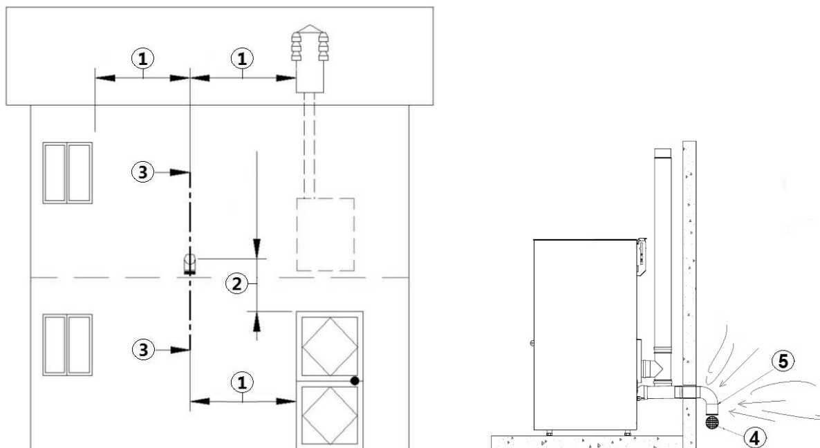
Fig. 11 - Presa d'aria per installazione a camera stagna
